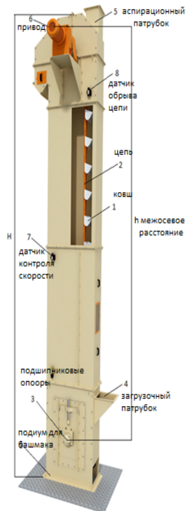
Рисунок цепного элеватора
