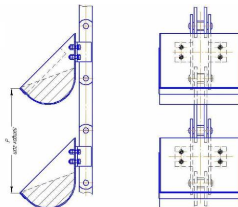
Пластинчатая цепь
