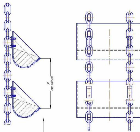
Круглозвенная цепь
